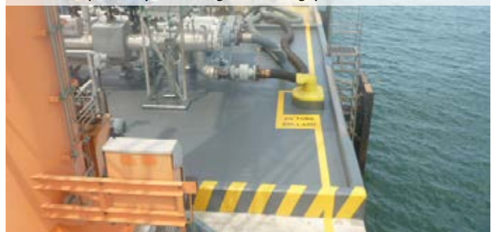
► Rutschfest und 1A-chemikalienfest - PROGUARD CN-1M für Öltransport-Jetty auf Jurong Island / Singapur
